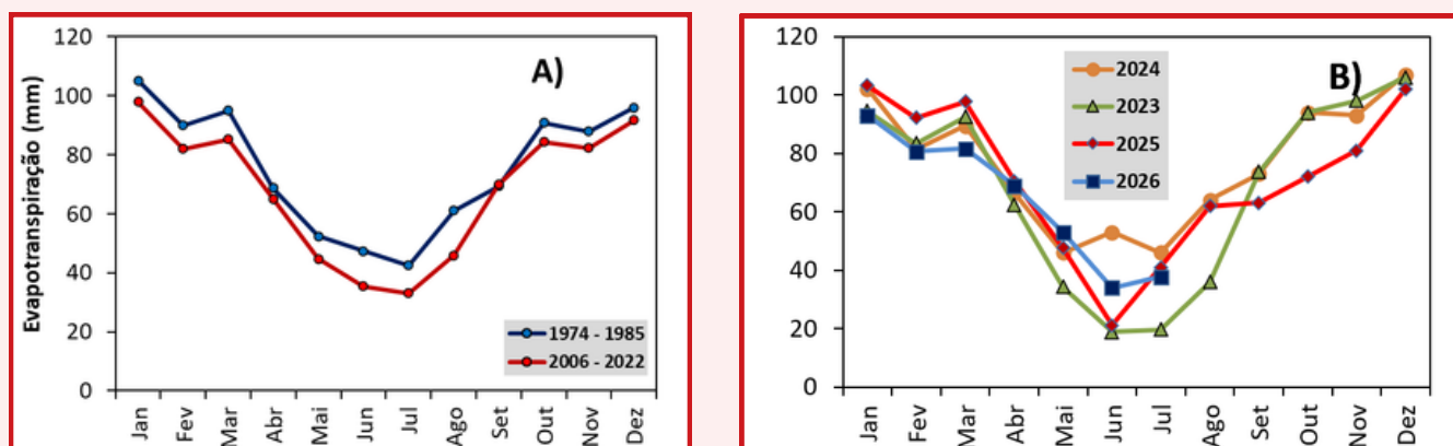
Figura 5: Evapotranspiração potencial mensal ( \text{mm mês}^{-1} ) das médias históricas de 1974-1985, 2006-2022 (A) e dos anos 2023, 2024, 2025 e 2026 (B) para a região do Sul de Minas, Muzambinho.
