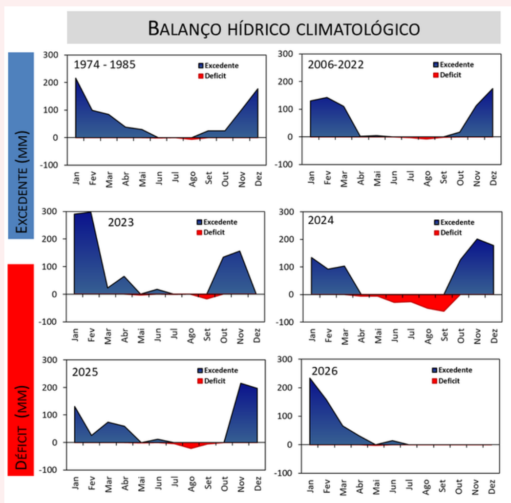
Figura 8: Balanço hídrico mensal (THORNTHWAIT E MATHER, 1955) no período de 1974-1985, 2006-2022, para os anos de 2023, 2024, 2025 e 2026 para a região do Sul de Minas, Muzambinho.
